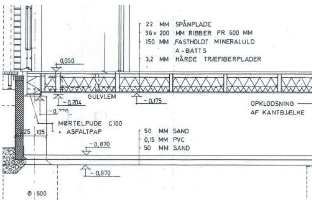
Figur 4. Opbygning af krybekælder bund og etageadskillelse.
