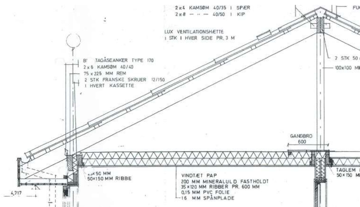
Figur 5. opbygning af tag- og loftkonstruktion med B6 bølge-eternit.
