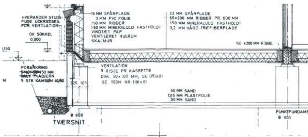
Figur 3. Snit af sokkel/fundaments-opbygning.
