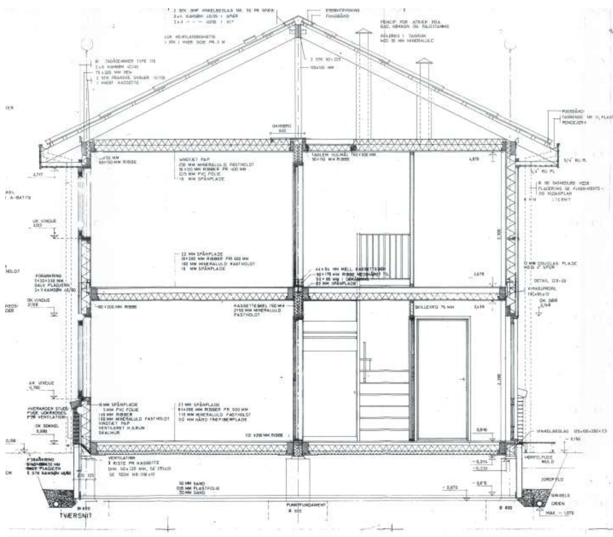
Figur 2. Tversnit af 2-etagers bolig.
